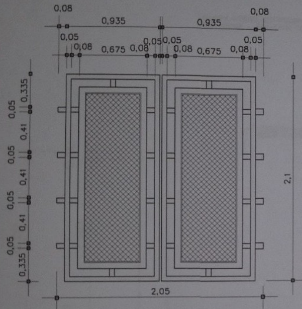
DET. PT1 ESC. 1:20
