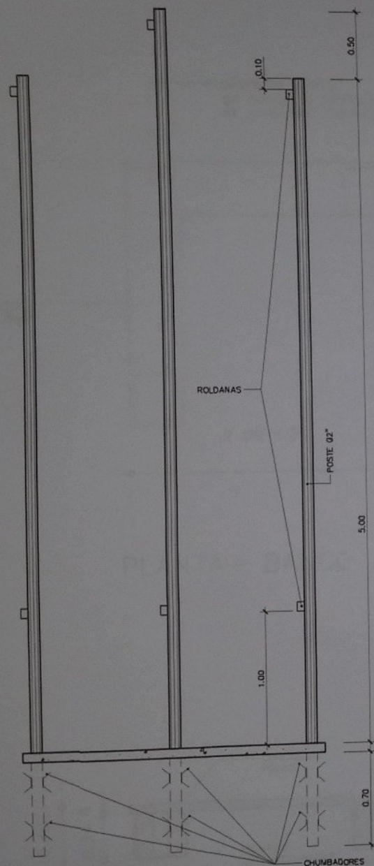
MASTROS DE BANDEIRAS DET. VISTA
