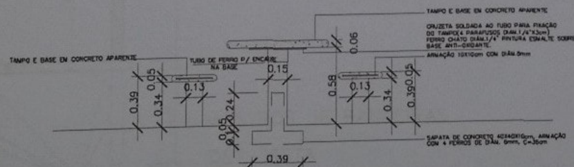
CORTE TRANSVERSAL
