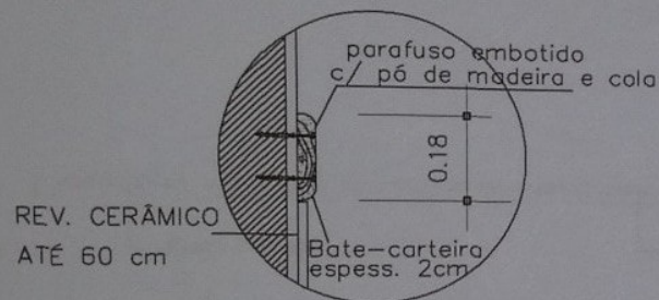
DET. BATE-CARTEIRA ESC. 1:2
