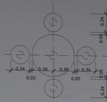
PLANTA MESA COM BANCOS DA PRAÇA
