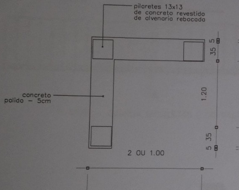
PLANTA - BANCO
