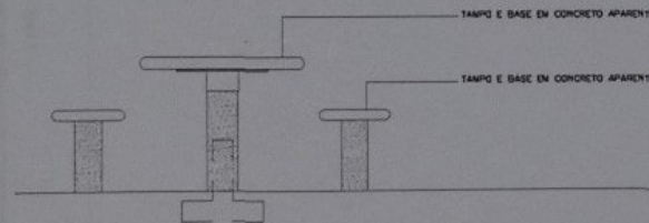
VISTA
