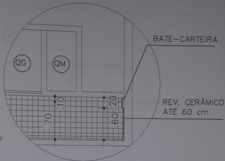
VISTA PAREDE QUADRO
