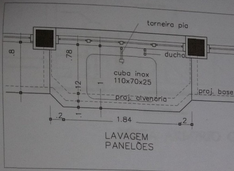
VISTA SUPERIOR BANCADA ESC. 1: 20
