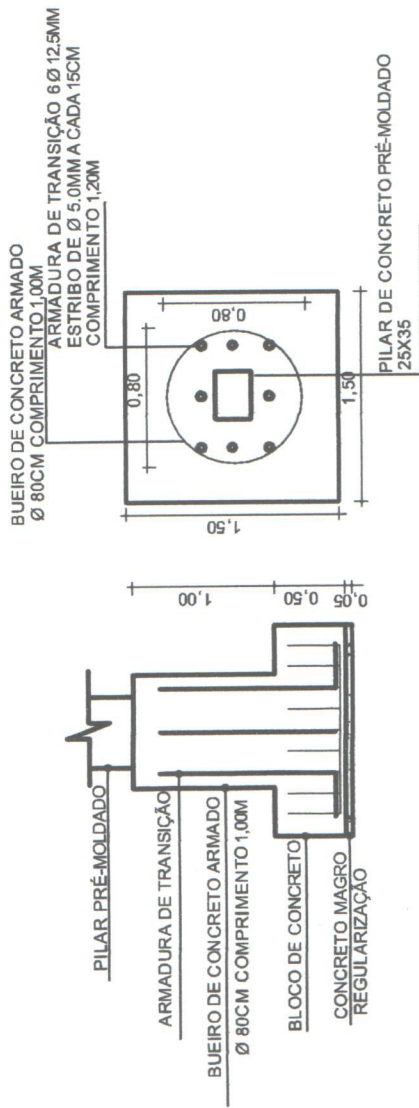
Detalhamento Bloco de Fundação Esc.: 1/50
