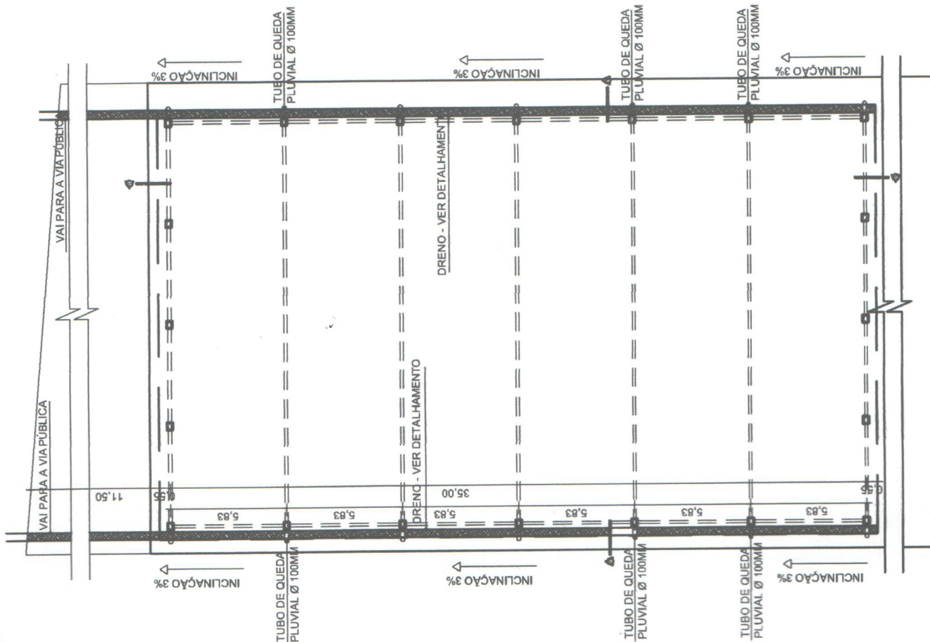
Planta Baixa - Drenagem Esc.: 1/250
