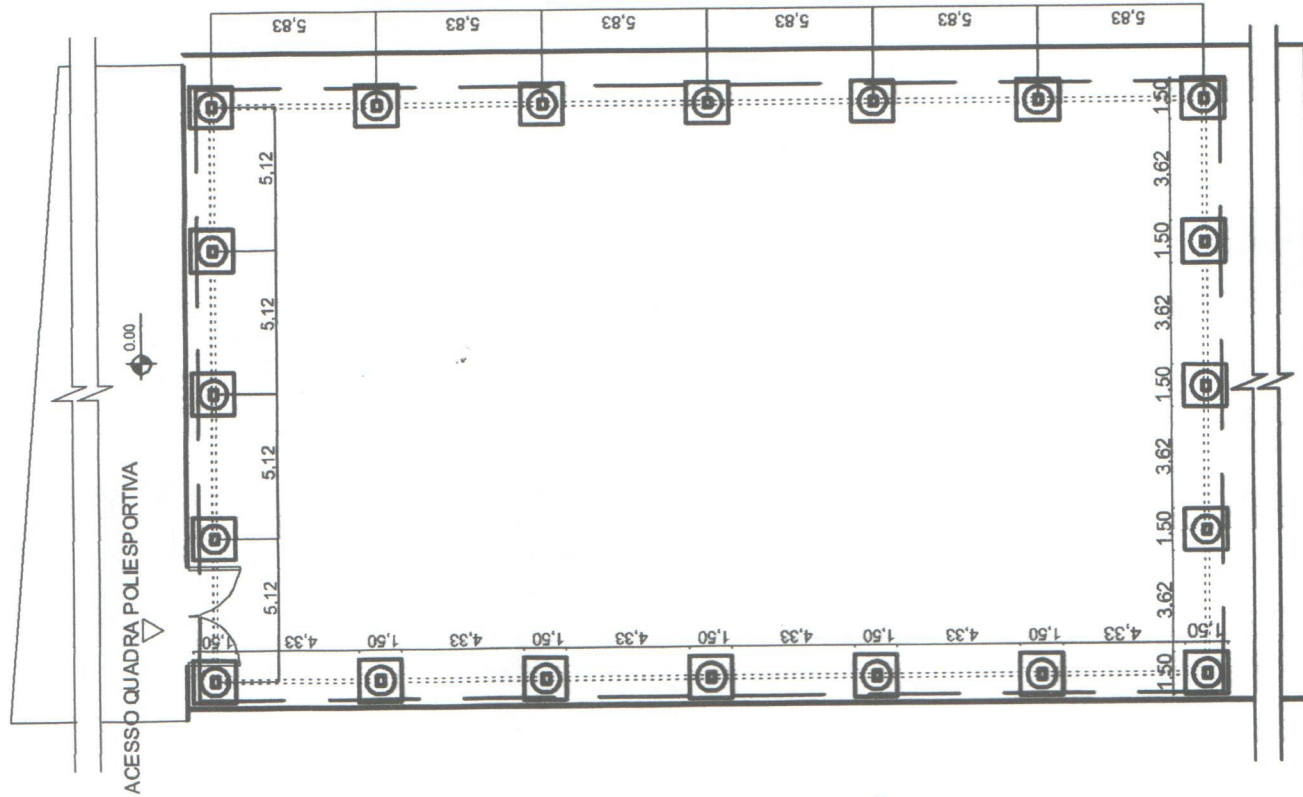
Projeto de Infra-estrutura Esc.: 1/250
